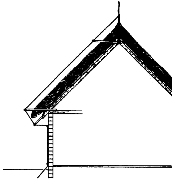
Fig. 3:11 Lightning conductor.
